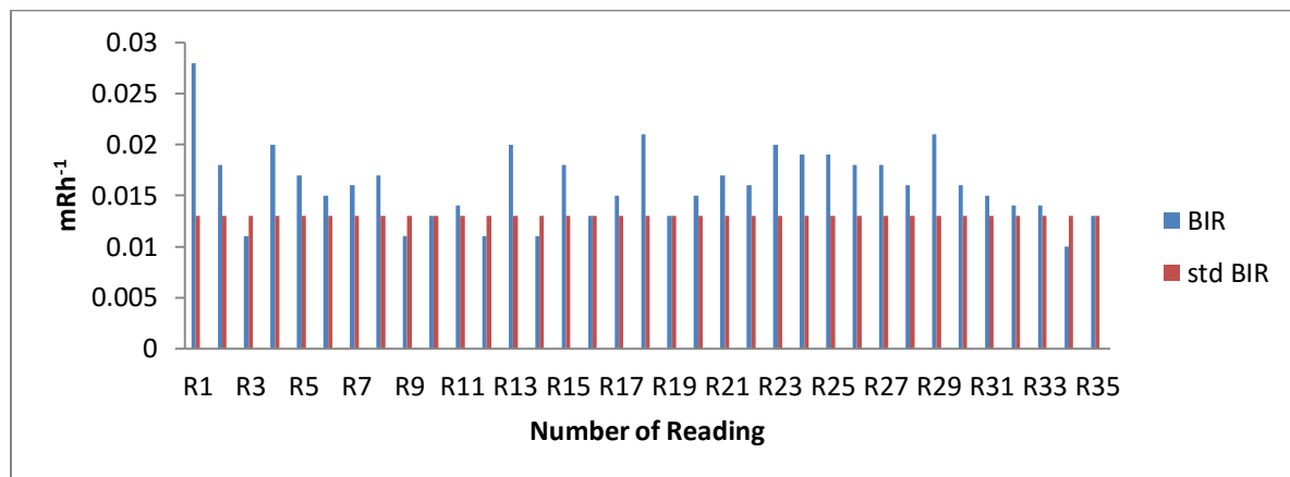
Fig. 2: Comparison of standard BIR and measured BIR
